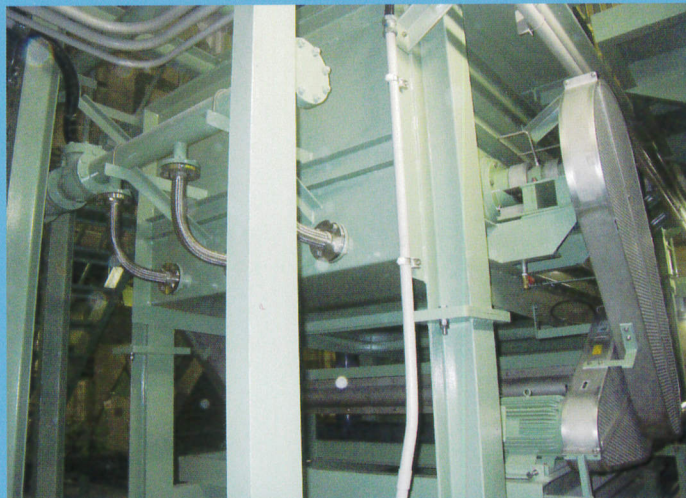
スクリーンかす洗浄装置
