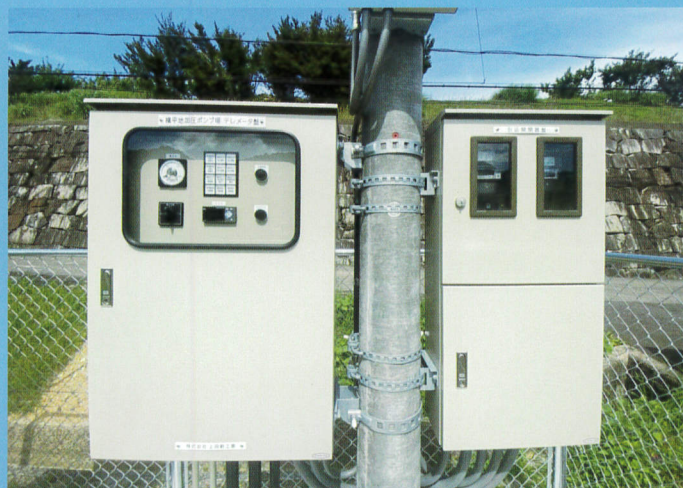
テレメータ盤・引込開閉器盤
