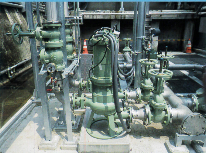
しき移送ポンプ(汚水しき移送装置)
